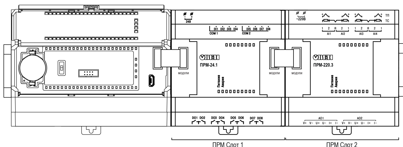
Рисунок 6.20 – Расположение модулей расширения на шине
