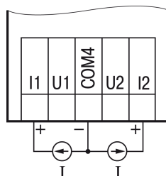
Рисунок 6.12 – Подключение датчиков с выходом в виде тока
