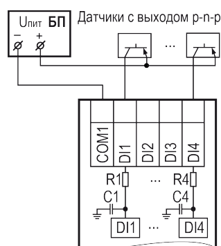
Рисунок 6.5 – Подключение к входам типа «Д» датчиков с выходом p-n-p
