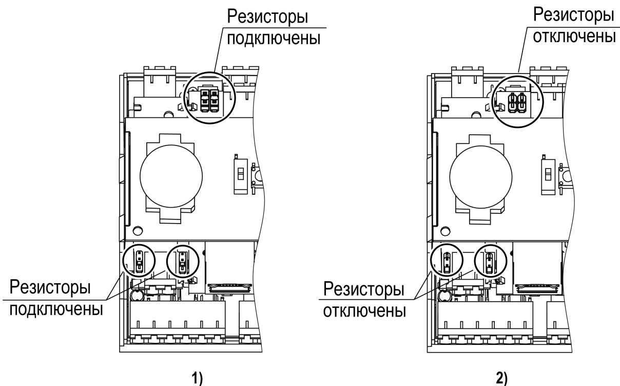
Рисунок 6.23 – Положение перемычек для встроенного интерфейса RS-485 и платы ПР-ИП485: 1) подтягивающие резисторы подключены, 2) подтягивающие резисторы отключены
