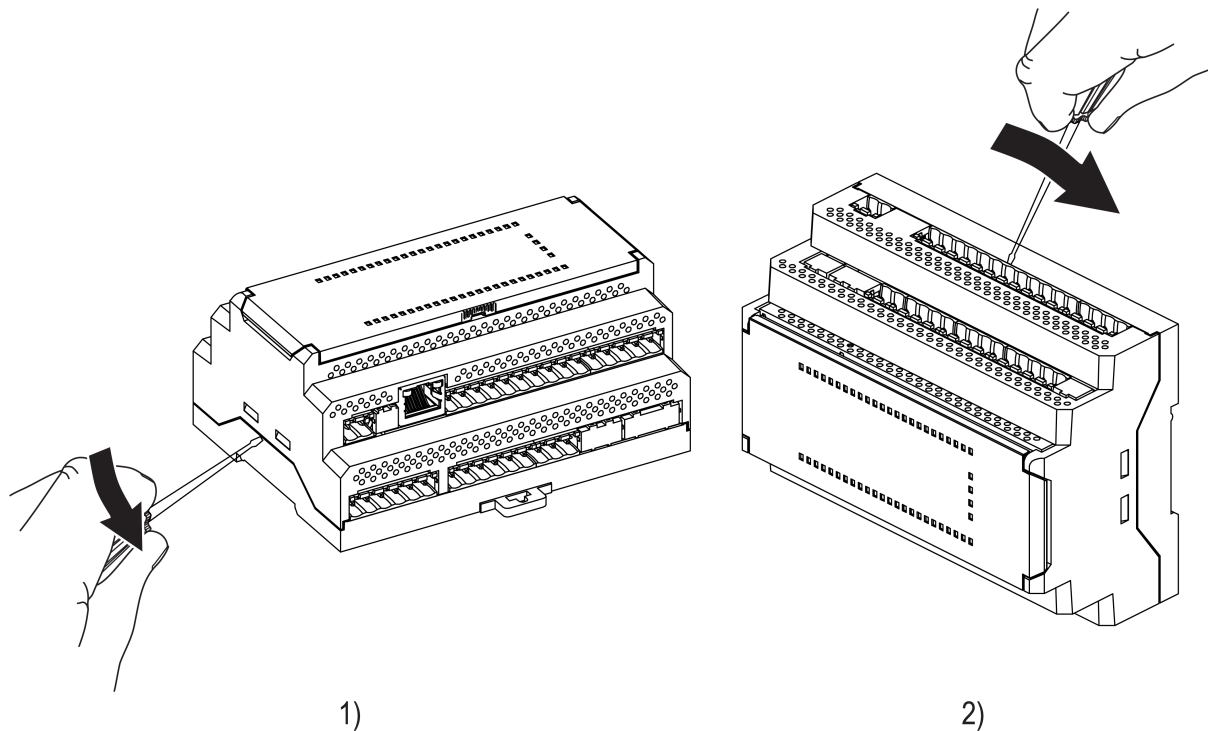
Рисунок 8.2 – Снятие верхней крышки
