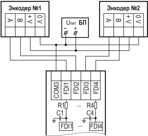
Рисунок 6.8 – Схема подключения АВ энкодеров
