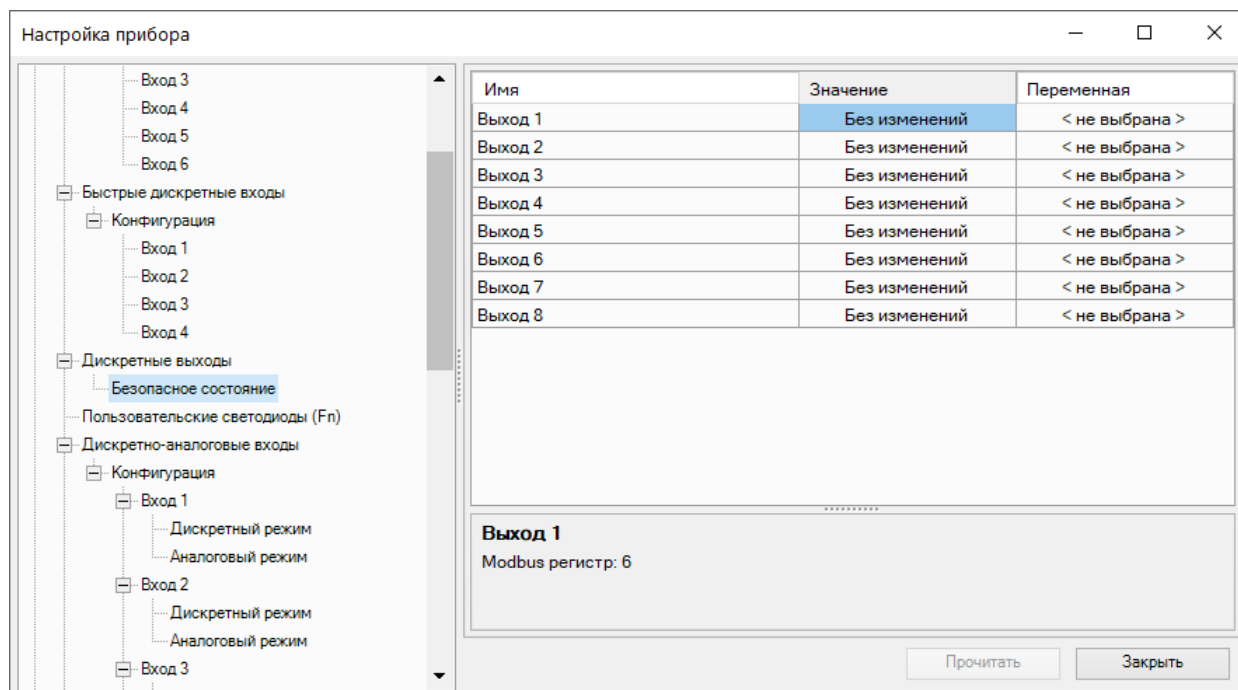
Рисунок 4.11 – Настройка безопасного состояния дискретных выходов прибора
