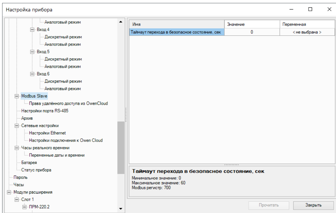
Рисунок 4.23 – Настройка таймута
