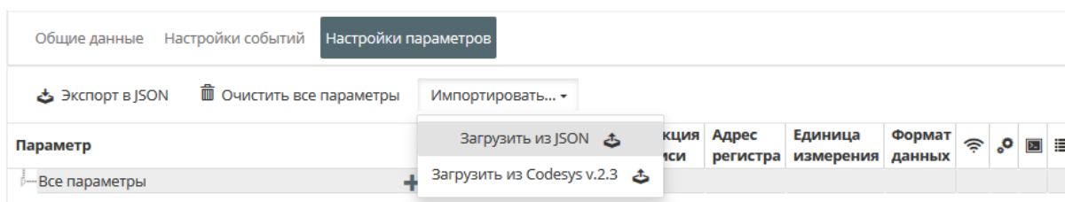
Рисунок 4.26 – Импорт параметров
