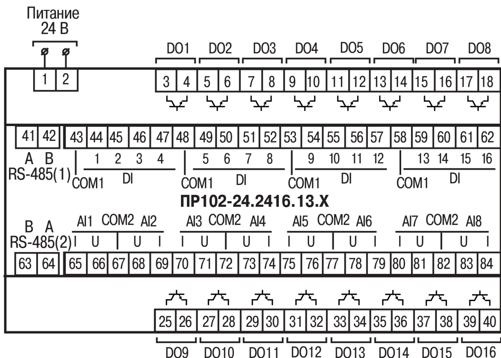
Рисунок А.4 – Расположение контактов для ПР102-24.2416.13.X
