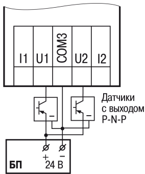
Рисунок 6.5 – Схема подключения к универсальным входам, работающим в дискретном режиме трехпроводных дискретных датчиков, имеющих выходной транзистор р-п-р-типа с открытым коллектором
