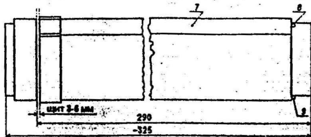
Рис.1. Габаритные и установочные размеры
