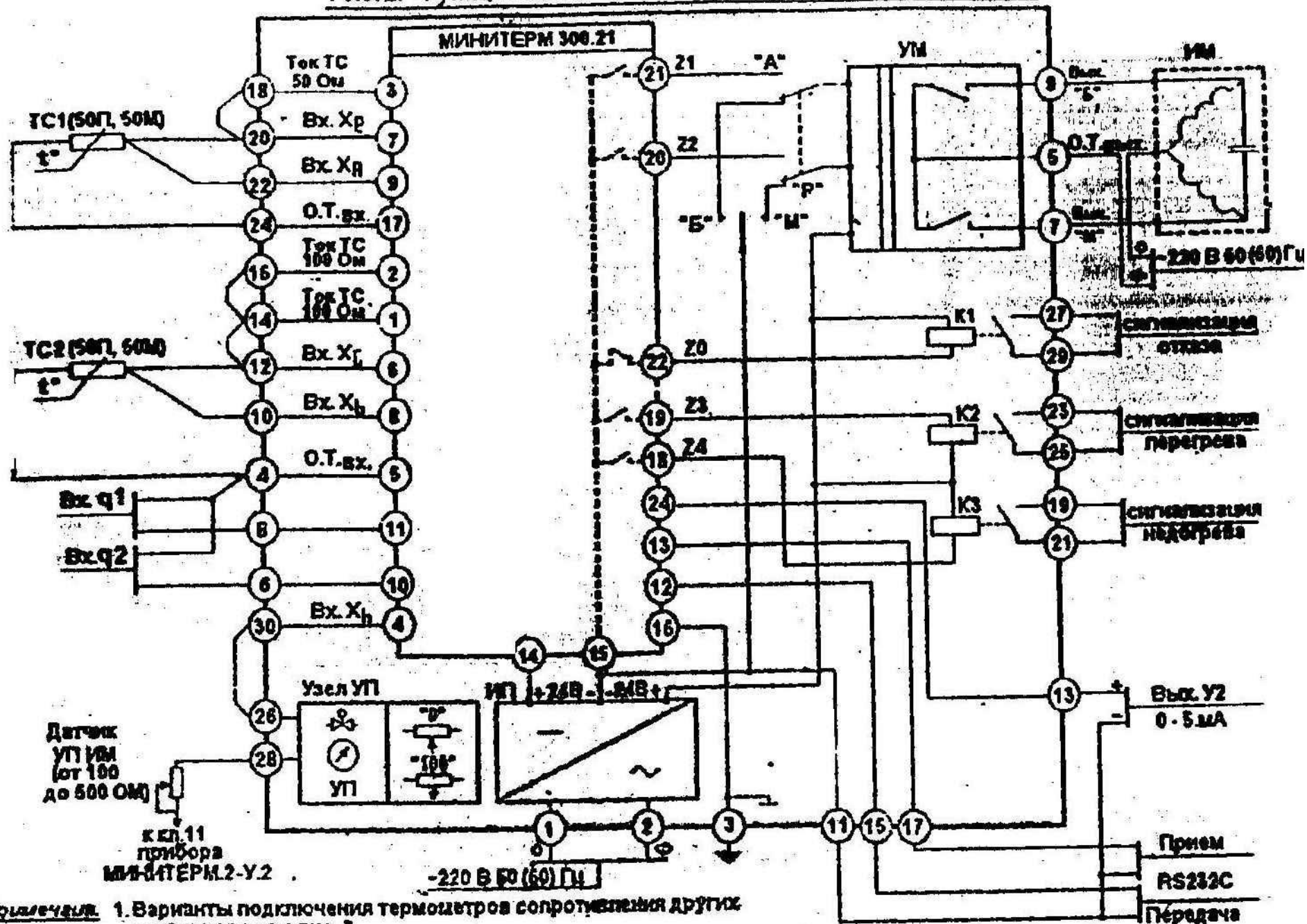
Рис.2. Функциональная схема прибора МИНИТЕРМ.2 - у.2
