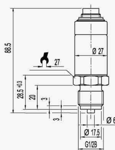
Образцовый преобразователь CPT6210
