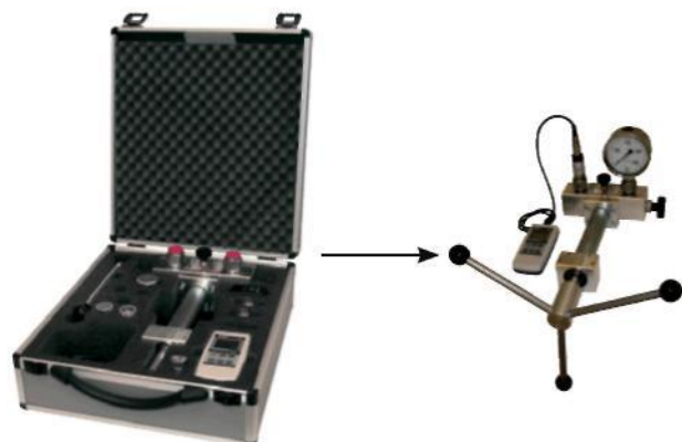
Базовое исполнение, включает гидравлический источник создания опорного давления
