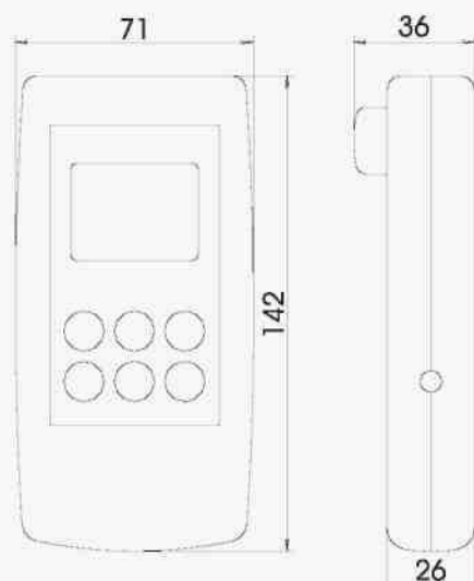
Цифровая консоль CPH6210
